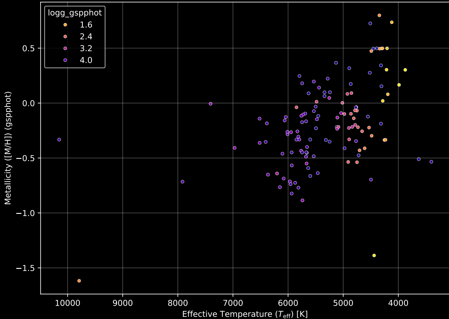
APOGEE DR17 Field: [278-37-O_TESS] Stellar Population Parameters (n= 126)
